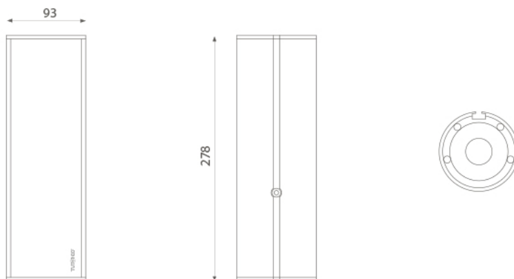
OLI C2 Dimensions: H278 x Ø93 mm
