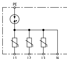
Schema di principio DG TT 5 275
