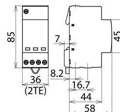
Dimensioni DG TT 5 275
