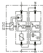
Schema di principio DG M TT 2P ACI 275 FM
