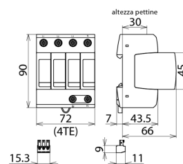
Dimensioni DG M TT 275 FM
