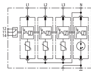
Schema di principio DG M TT 275 FM
