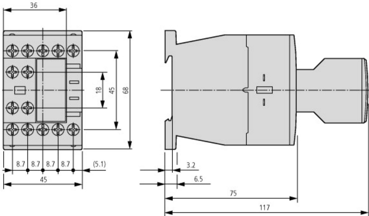
Contattori con modulo contatti ausiliari
