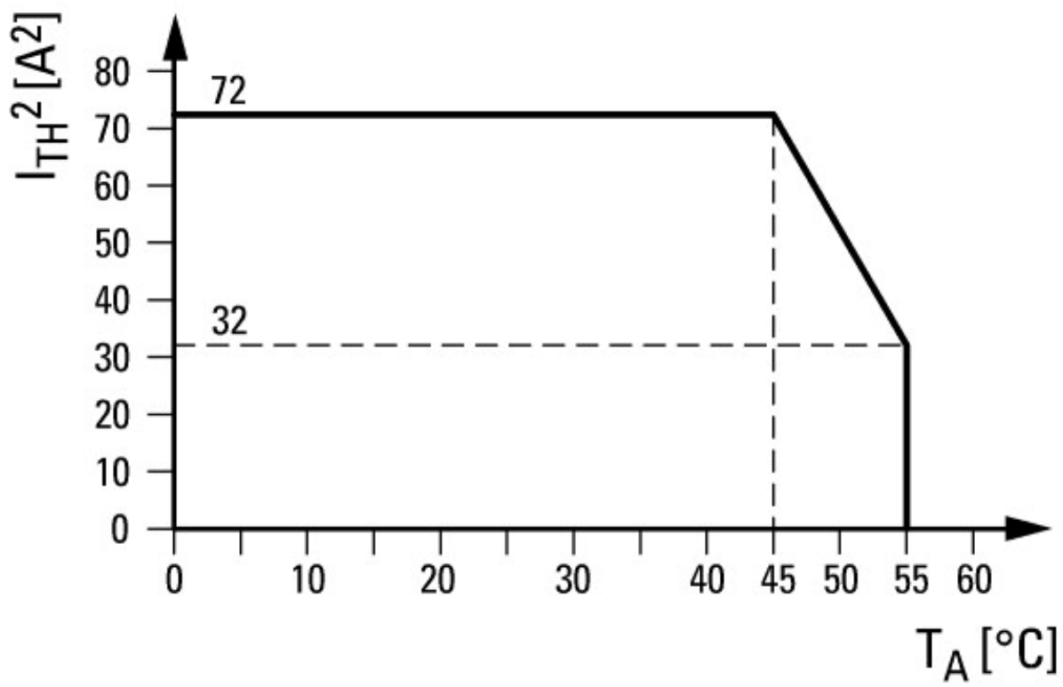
Curva di derating
