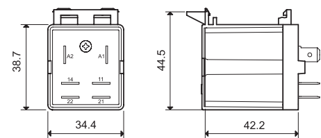
065.08 con relè
