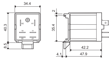
065.07 con relè
