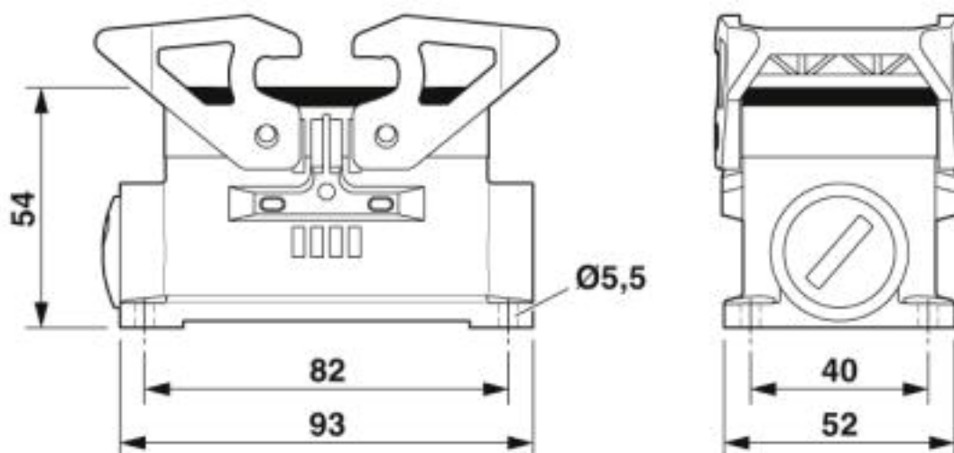
Disegno quotato
