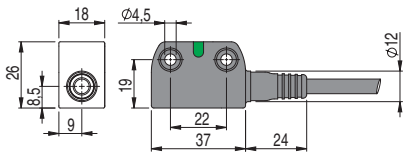
Sensore ST G••••N• con cavo
