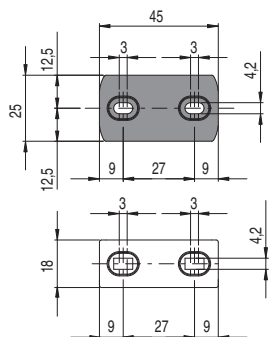
Azionatore SM D•T
