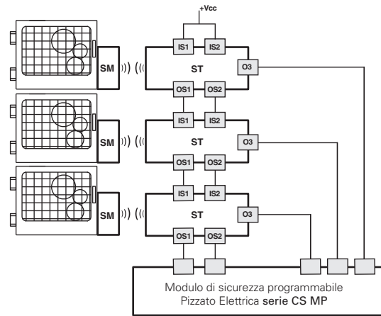
Collegamento con modulo di sicurezza programmabile
