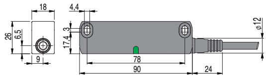
Sensore ST H••••N• con cavo
