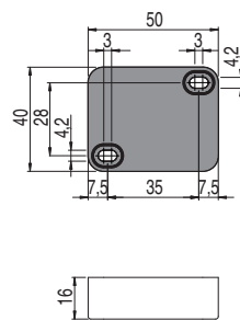
Azionatore SM E•T
