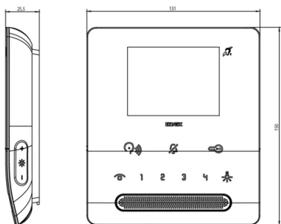
Vista ingombri
