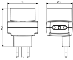
Vista ingombri
